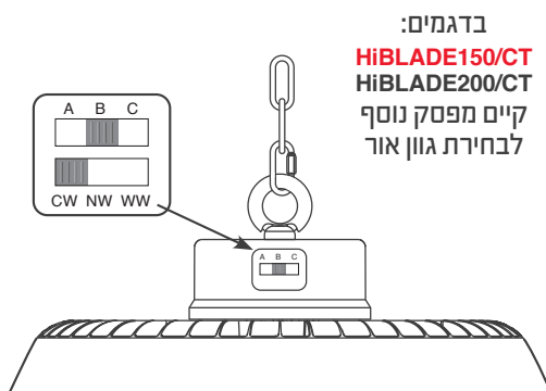
HiBLADE200
