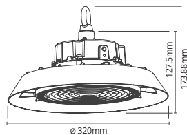
200W HiBLADE200
